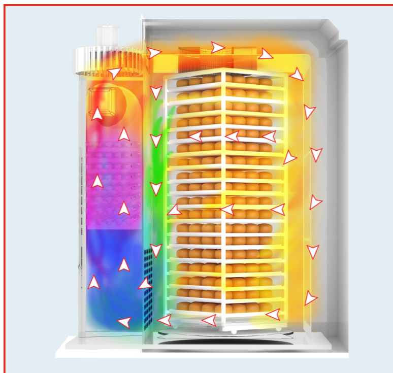
Схема движения воздуха в ротационной печи «Муссон-ротатор» модель 99/11-01
